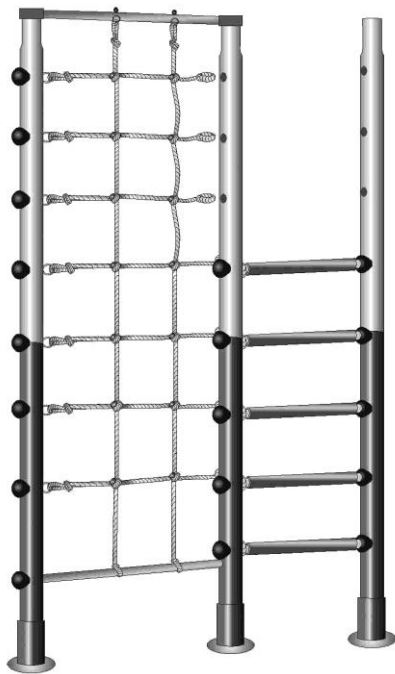
Рис.3 Сборка лестницы со стойкой
